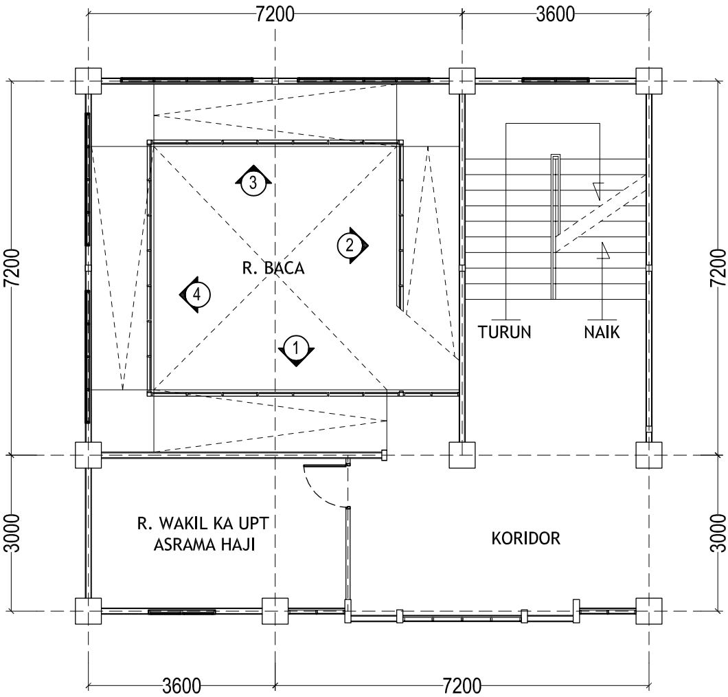
1 ARS DENAH RENCANA R. BACA LT. 2 SKALA 1 : 100
