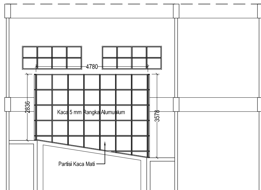
1 ARS TAMPAK 3 SKALA 1 : 100
