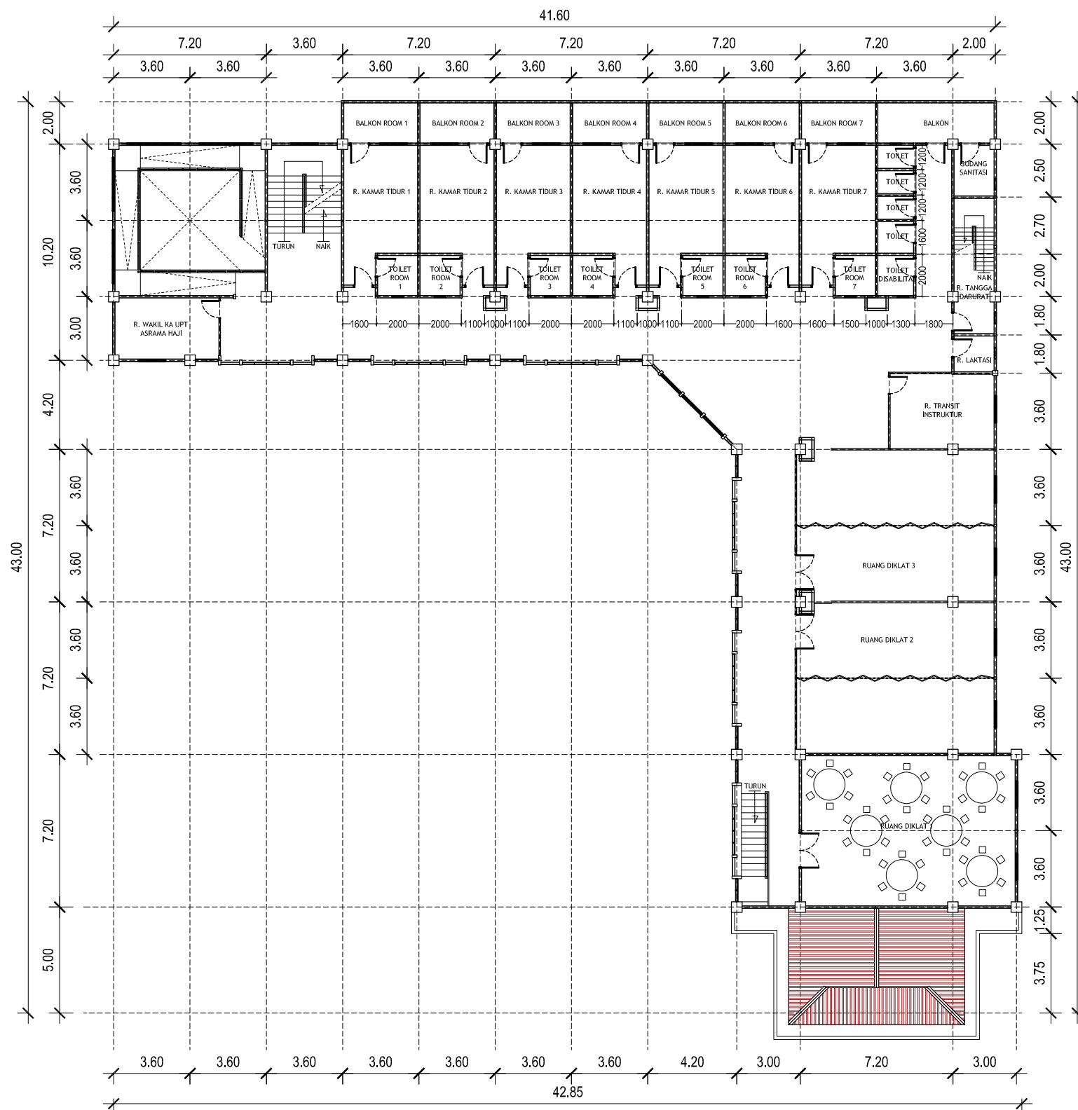
1 DENAH LANTAI 2 RENCANA ARS SKALA 1 : 250
