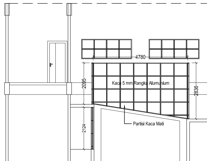
1 ARS TAMPAK 4 SKALA 1 : 100
