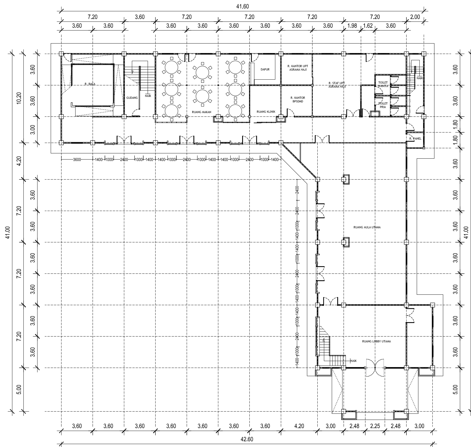
1 DENAH LANTAI 1 RENCANA ARS SKALA 1 : 250
